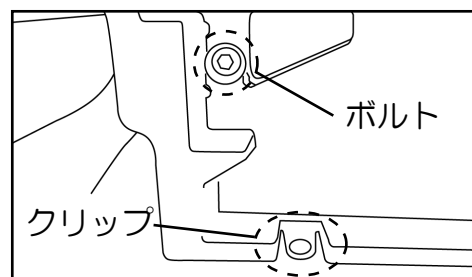
図 B. サイドトリム下部のクリップ側面のボルトを取り外す
