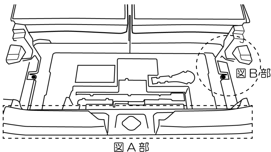
図 A. スカッフプレートを持ち上げ取り外す
